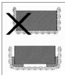
Figura 10. Uso de cantoneras.
